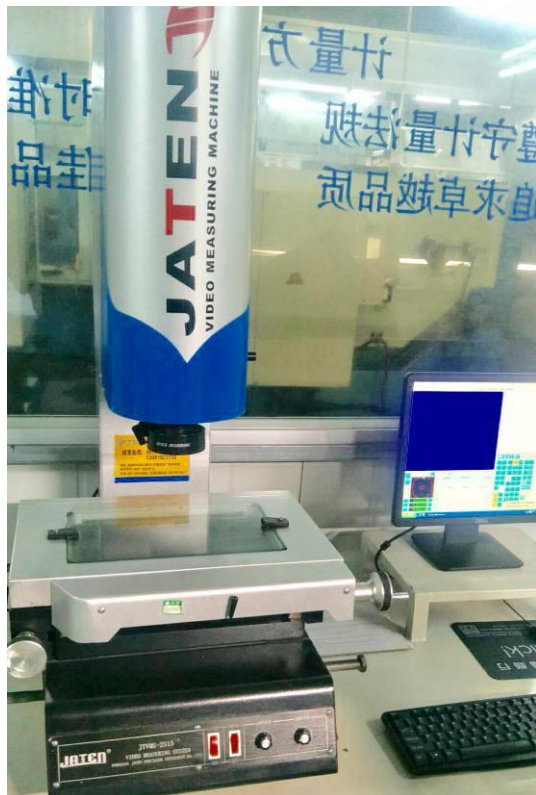
Видеоизмерительная машина
